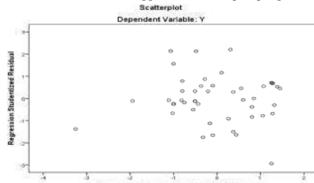
Sumber: (Olai Data SPSS 22, 2026) Gambar 3. Uji Heterokedastisitas
